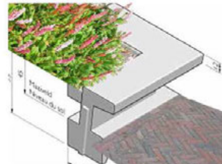
-8- Bloembakken van beton eventueel met zitrand, voor vaste beplanting.
