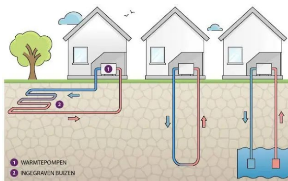
Afb. 2: Aardwarmte: voorbeeld van een onder de grond geplaatste lus.
